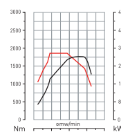
DTI 11 - 380 PK
