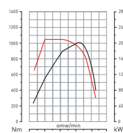
DTI 8 - 280 PK
