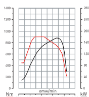
DTI 5 - 240 PK
