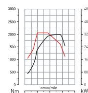
DTI 11 - 430 PK
