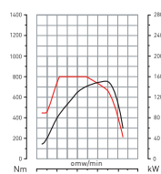
DTI 5 - 210 PK
