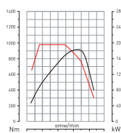
DTI 8 - 250 PK
