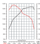
NGT 9 - 320 PK
